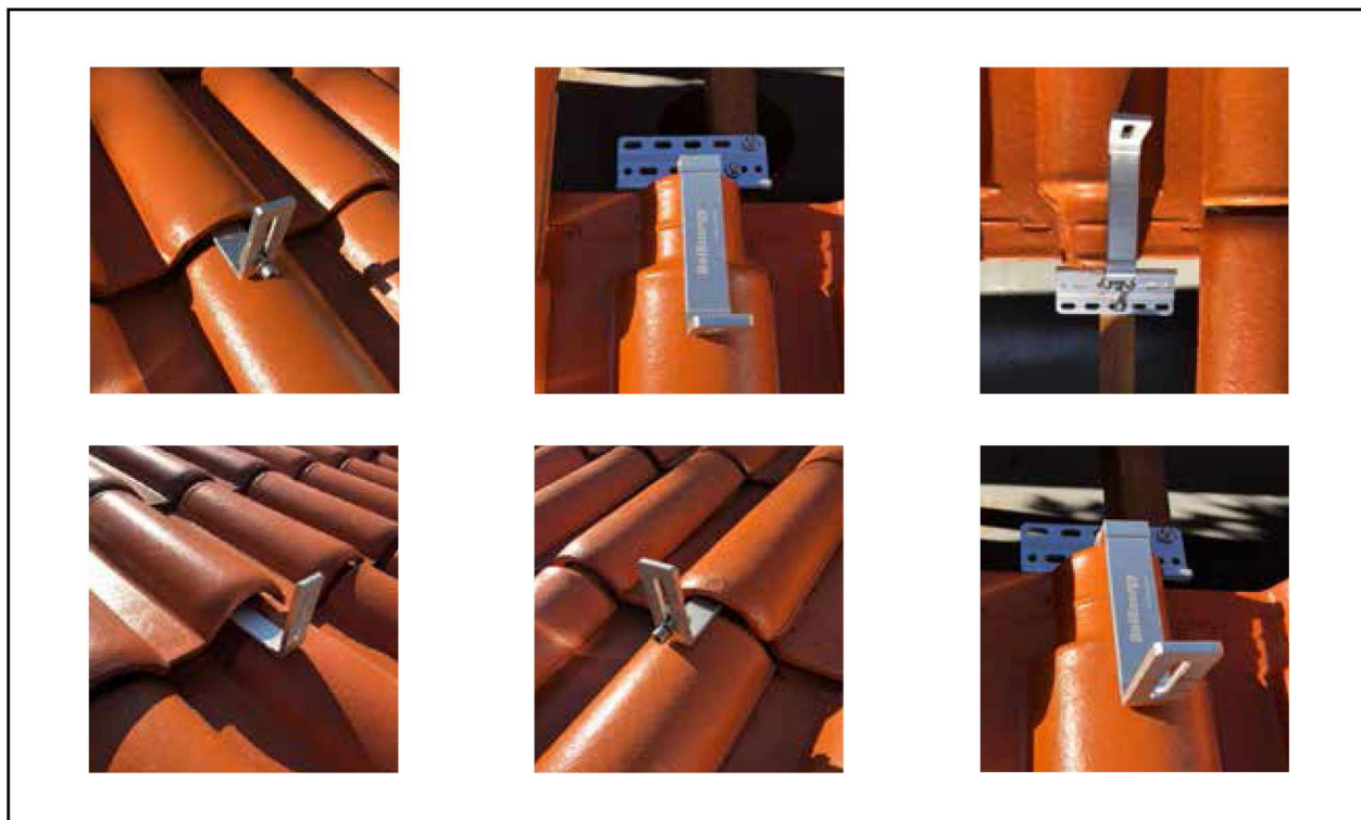
Figura 10 - Aplicação do suporte
