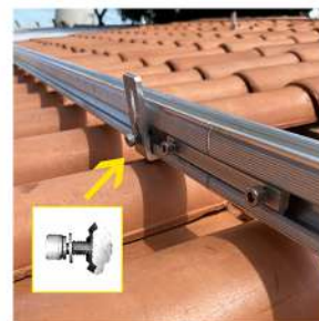
Figura 4 - Encaixe do perfil
