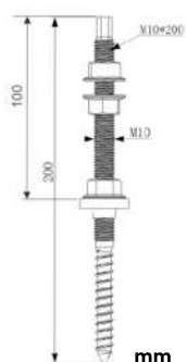
Figura - Hastes solares
